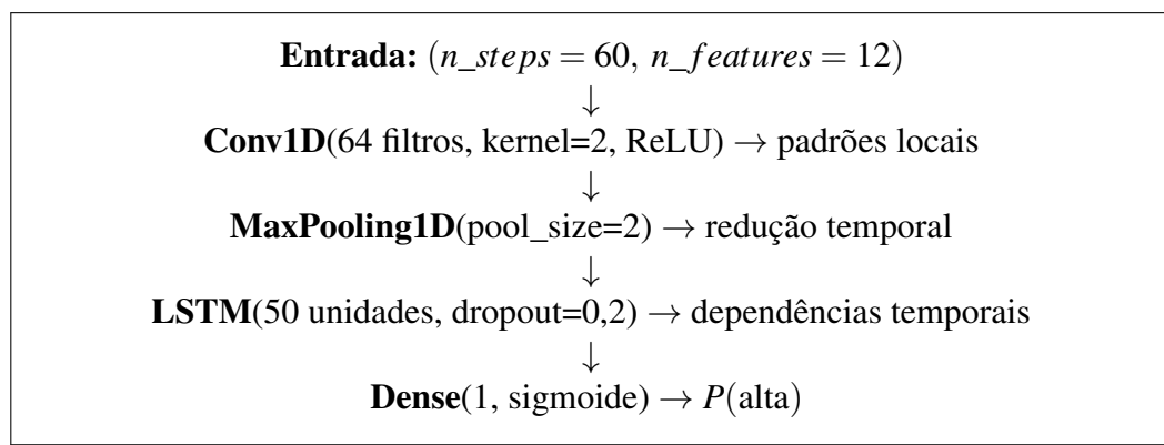
Figura 9 – Arquitetura do modelo híbrido CNN-LSTM (proposta). Fonte: o autor, a partir de cnn_lstm_model.py .
